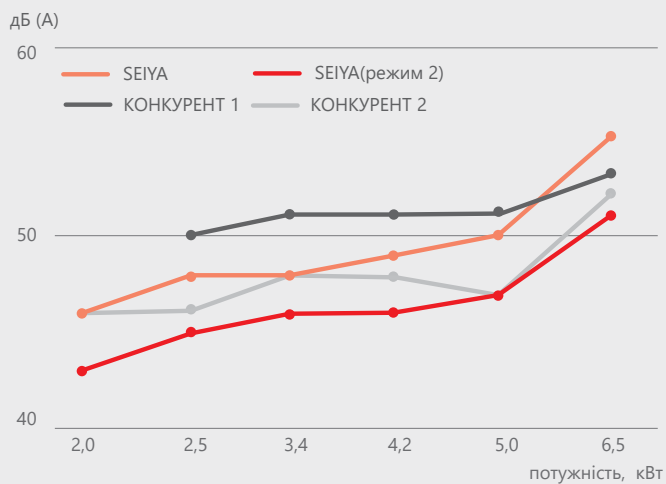
Рівень шуму зовнішніх блоків
