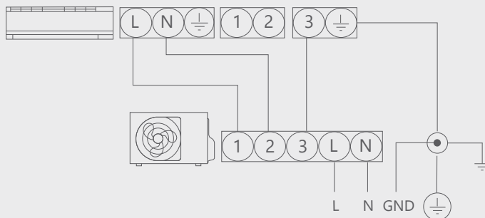
Електрична схема (опціональна)
