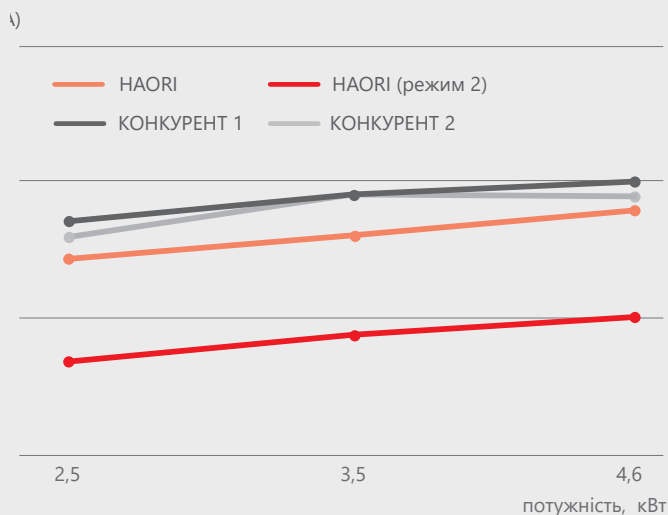
Рівень звукового тиску зовнішніх блоків дБ(А)
