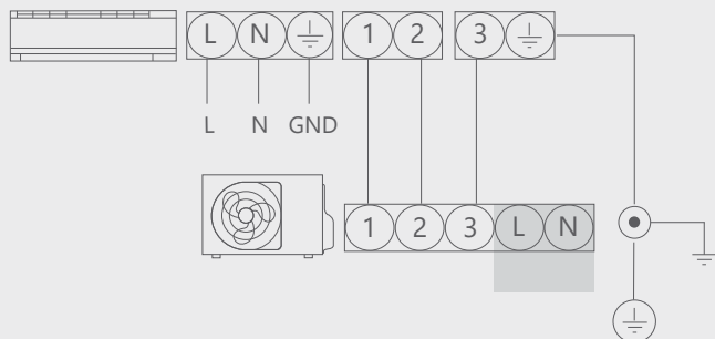
Електрична схема (рекомендована)
